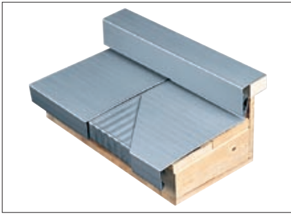
Detailanschnitt Gesimsabdeckung
